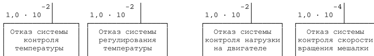
Рисунок 8-1. Пример дерева отказов для химических реакторов
